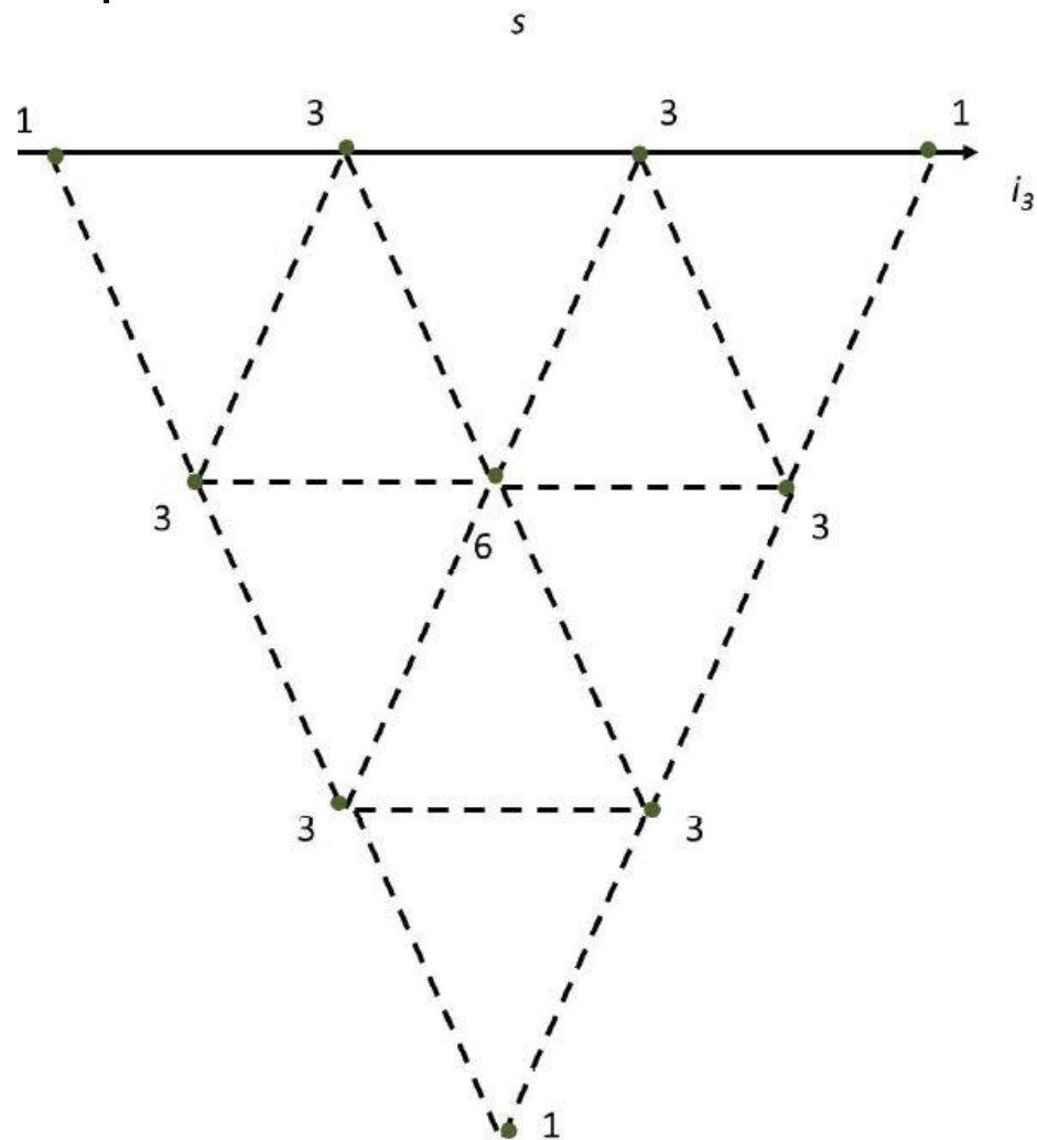
u, d, s + 2 kvarka
