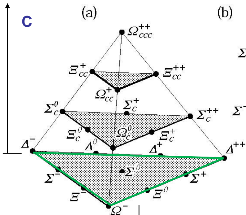
dekuplet u, d, s barionov
