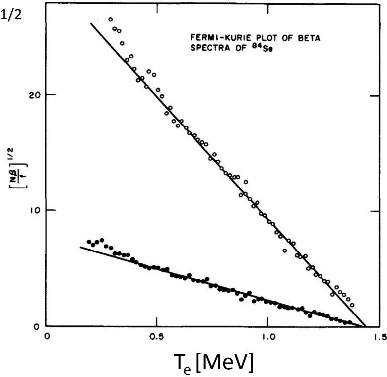
Fermi-Kurie graf
