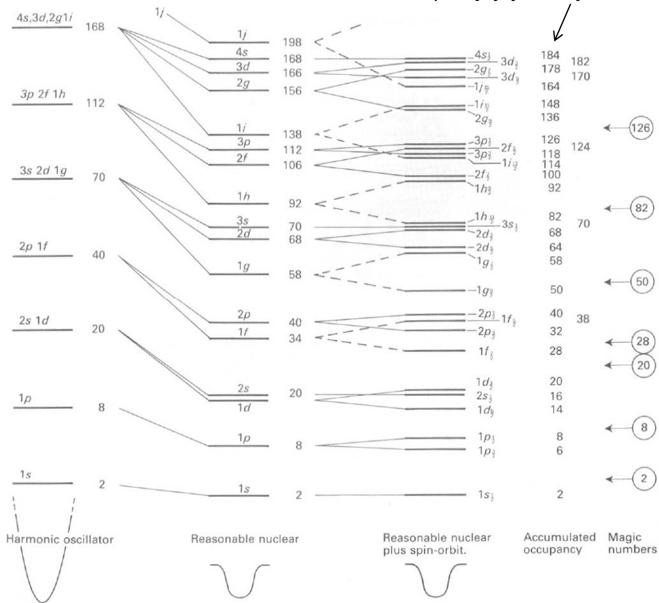
Energijski nivoji v različnih približkih potenciala
