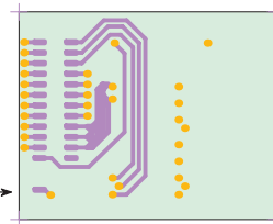
Bottom Layer
