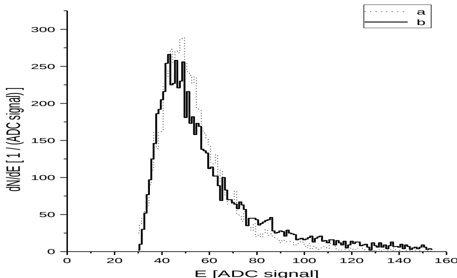
Slika 3.7: Izmerjeni spekter odložene energije v detektorju (a.) in spekter, generiran po Landau-ovi porazdelitvi za minimalno ionizirajoče elektrone v siliciju (b.). Debelina aluminijaste plošče pri (a.) znaša 0 mm. Oba spektra sta normirana na enako število dogodkov.
