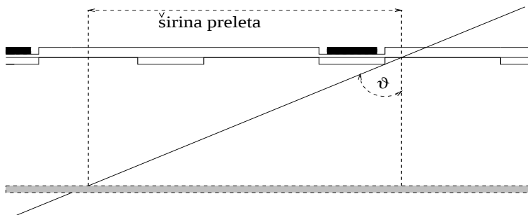
Slika 3.4: Prehod elektrona pod kotom.
