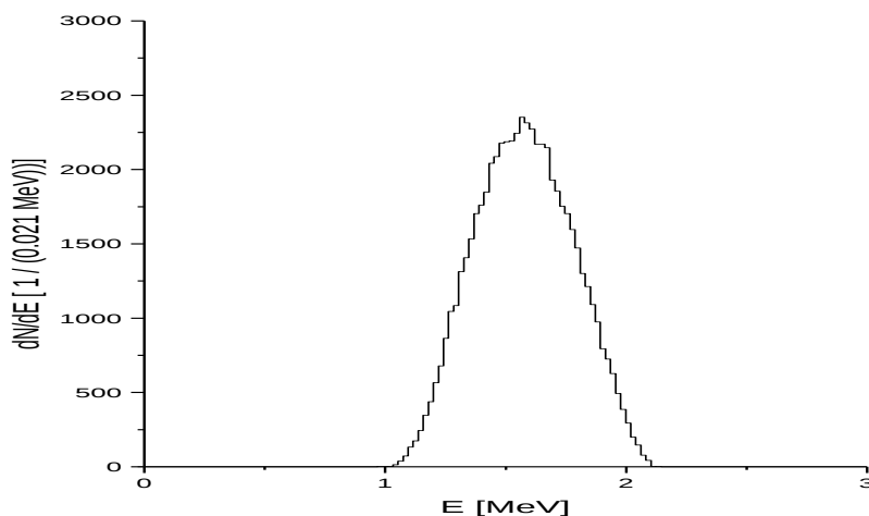
Slika 2.5: Spekter zaznanih elektronov pred vstopom v silicij. Debelina aluminijaste plošče je 1,4 mm.
