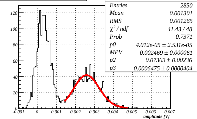
Amplitude, HV=1000V 200MHz
