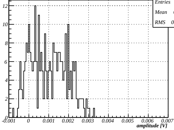
Amplitude, HV=1000V
