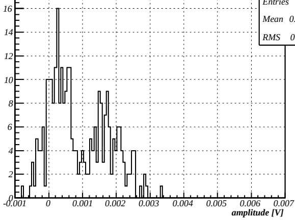
Amplitude, HV=800V
