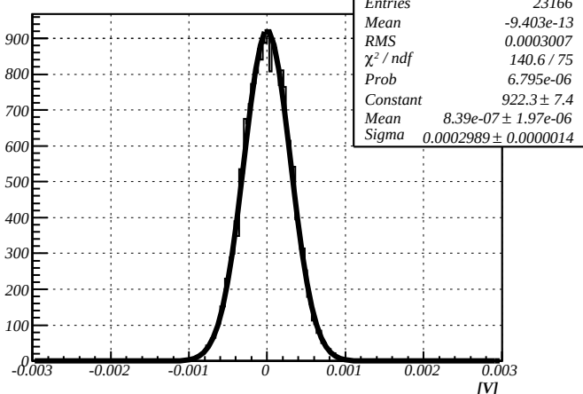
Noise, HV=0V
