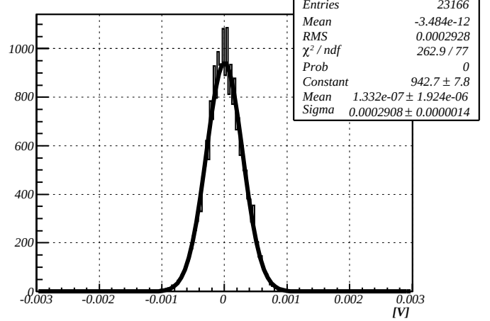
Noise, HV=800V
