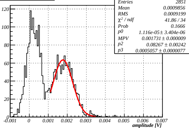
Amplitude, HV=1000V
