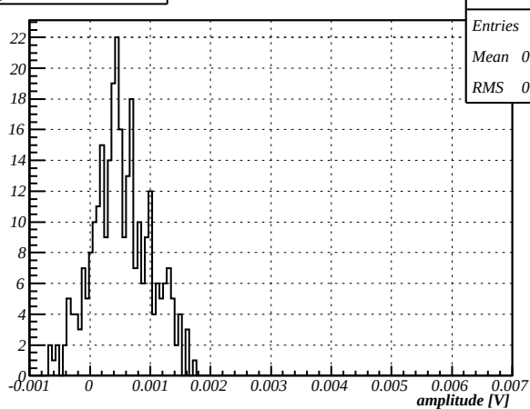
Amplitude, HV=-200V
