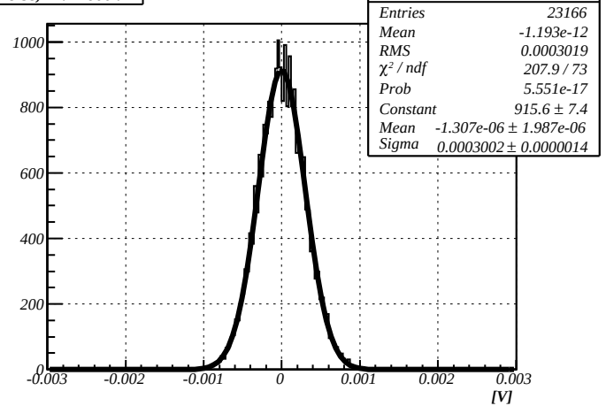
Noise, HV=-600V
