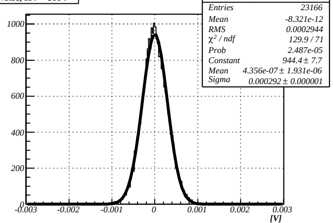
Noise, HV=-800V
