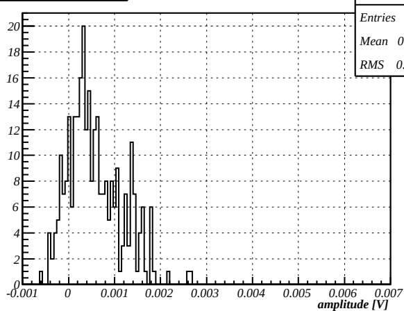
Amplitude, HV=-400V
