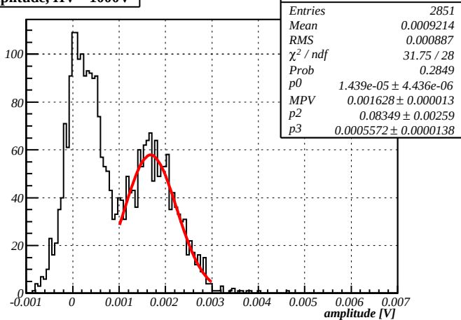
Amplitude, HV=-1000V
