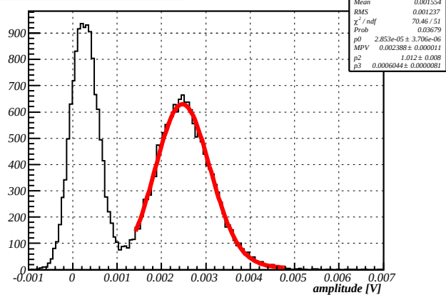
Amplitude, HV=1000V 200MHz
