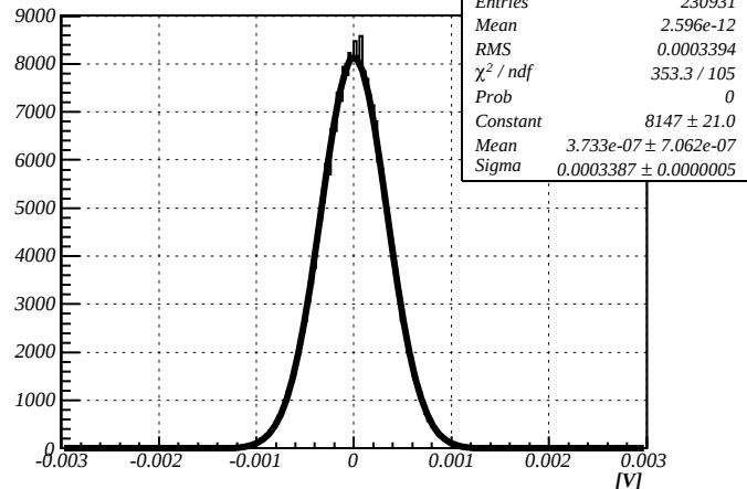
Noise, HV=-600V
