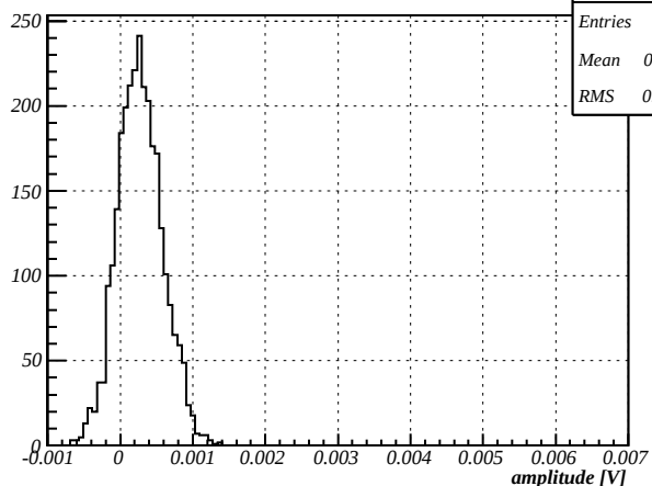
Amplitude, HV=-0V
