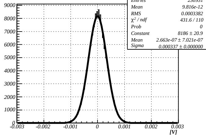
Noise, HV=-800V
