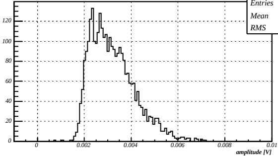
Amplitude, HV=1000V
