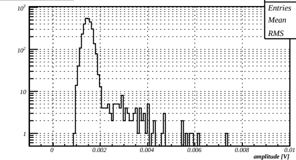
Amplitude, HV=1000V
