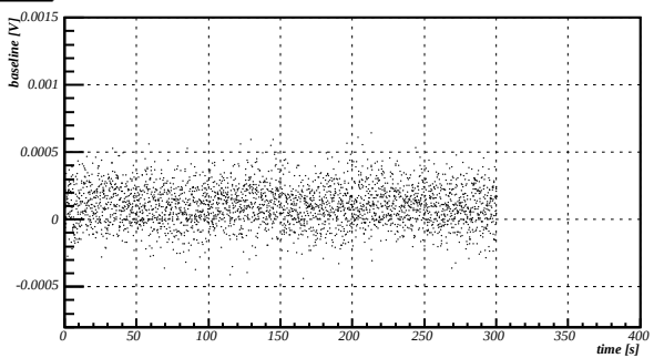
baseline
