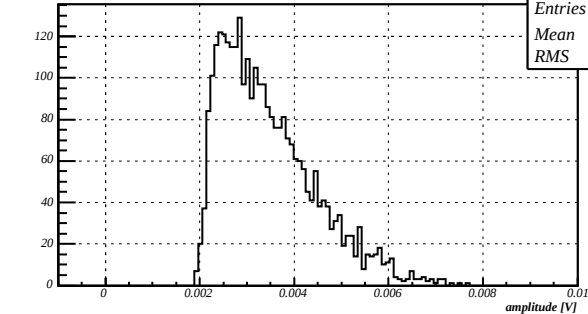
Amplitude, HV=1000V
