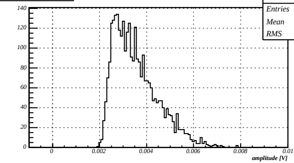
Amplitude, HV=1000V
