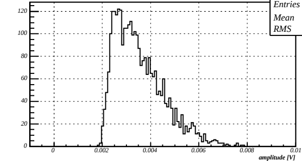
Amplitude, HV=1000V
