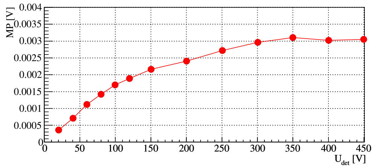
Signal(Q)
