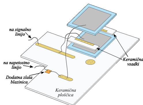
Slika 7.4: Levo: konfiguracija sestava z dvema diamantnima senzorjema. Desno: Slika senzorjev v detektorskem modulu.
