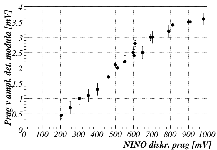
Slika 7.12: Korelacija med NINO diskriminacijskim pragom in pragom na skali amplitud vhodnega analognega signala. Slednje vrednosti so bile odčitane iz grafov kot so prikazani na sliki 7.11.
