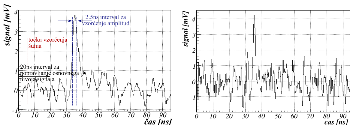
Slika 7.7: Tipičen časovni poteke signala zabeležen pri 200 MHz (levo) in 1 GHz (desno) frekvenčni pasovni širini na bralnem osciloskopu pri meritvah v laboratoriju s ^{90}\text{Sr} kot izvorom 1 MIP signalov.
