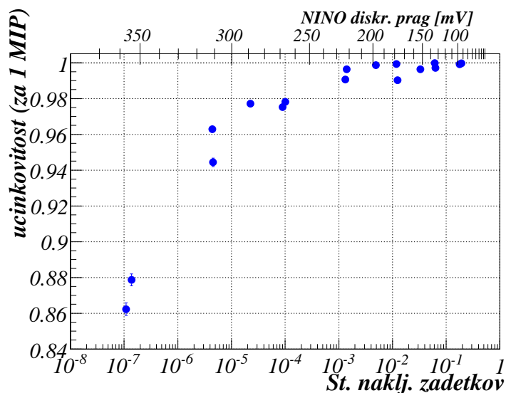
Slika 7.10: Ocenjena učinkovitost za detekcijo 1 MIP delca v odvisnosti od števila naključnih zadetkov (v enem detektorskem modulu) v časovnem intervalu med prehodoma dveh zaporednih gruč (25 ns), ki jo pričakujemo v ATLAS-u.
