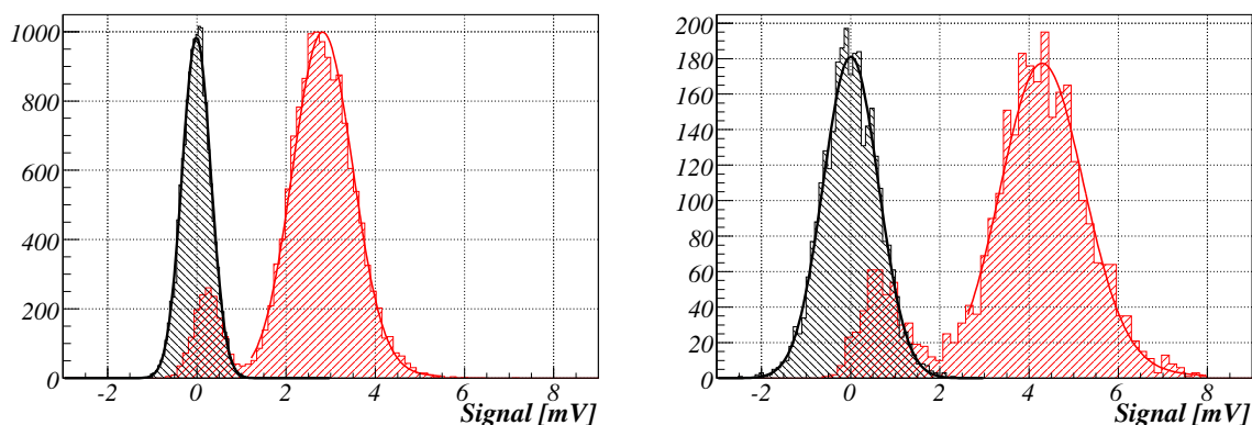
Slika 7.8: Porazdelitev šuma (črna) in amplitude (rdeča) za detektorski modul F402 izmerjen pri napetosti 1000 V (polje 2 \text{ V}/\mu\text{m} ) ter frekvenčni pasovni širini (levo) 200 MHz in (desno) 1 GHz na bralnem osciloskopu. Meritve so bile narajene s ^{90}\text{Sr} kot izvorom 1 MIP delcev.
