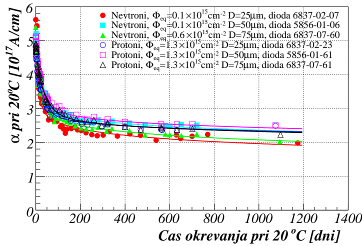
Slika 7.15: Časovni potek okrevanja (pri T_a=20^\circ ) zapornega toka za nekaj primerov obsevanih diod. Zaporni tok je naveden pri referenčni temperaturi T_r=20^\circ\text{C} . Črte predstavljajo rezultat prilagajanja funkcije 7.11.
