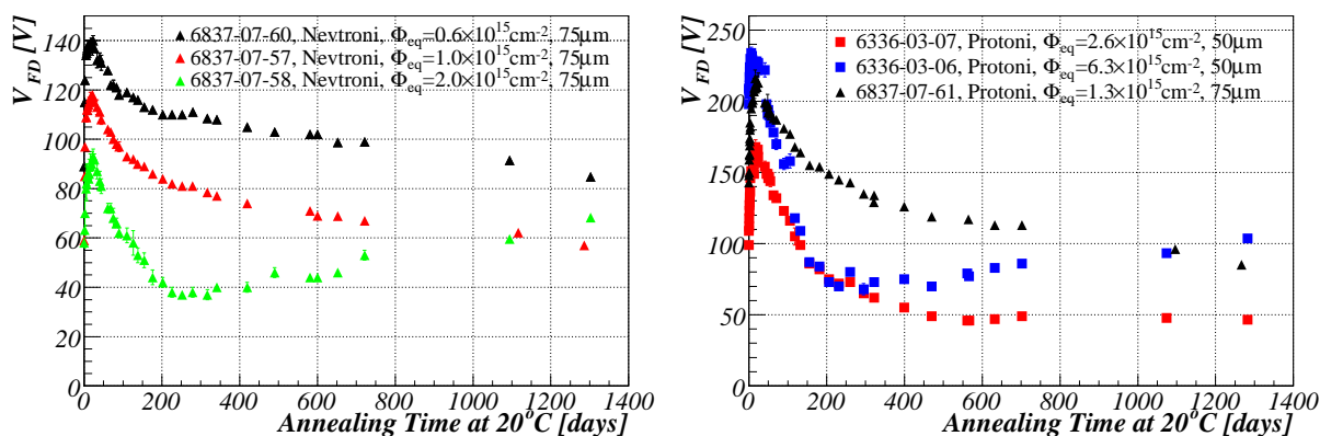
Slika 7.13: Izmerjene vrednosti V_{FD} skozi okrevanje pri 20^\circ\text{C} za epi diode obsevane z nevtroni (levo) in protoni (desno). Fluencia in debelina za vsako od diode so podane v legendi.
