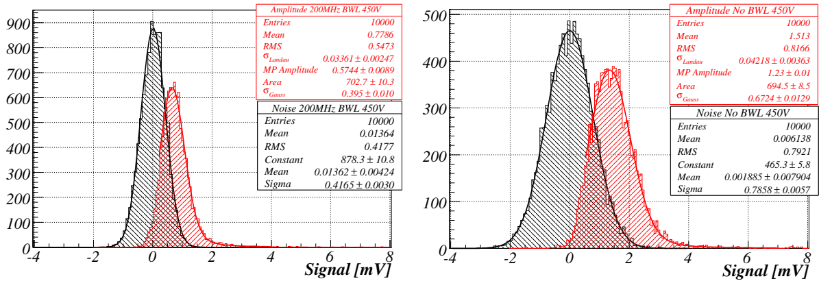
Slika 7.17: Porazdelitev amplitud (rdeča) in šuma (črna) izmerjena s 50 µm epi diodo pri zaporni napetosti 450 V ter 200 MHz (levo) oziroma 1 GHz frekvenčni pasovni širini na bralnem osciloskopu.
