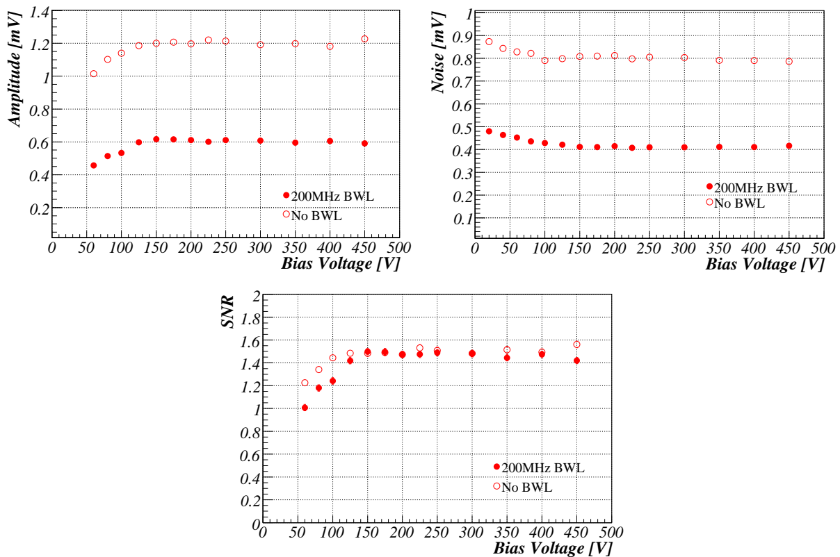
Slika 7.18: Odvisnost izmerjenih MP amplitud (levo), šuma \sigma_n (desno) ter razmerja signal–šum (spodaj) od zaporne napetosti na 50 µm epi diodi pri 200 MHz (polni simboli) ali 1 GHz (prazni simboli) na bralnem osciloskopu.
