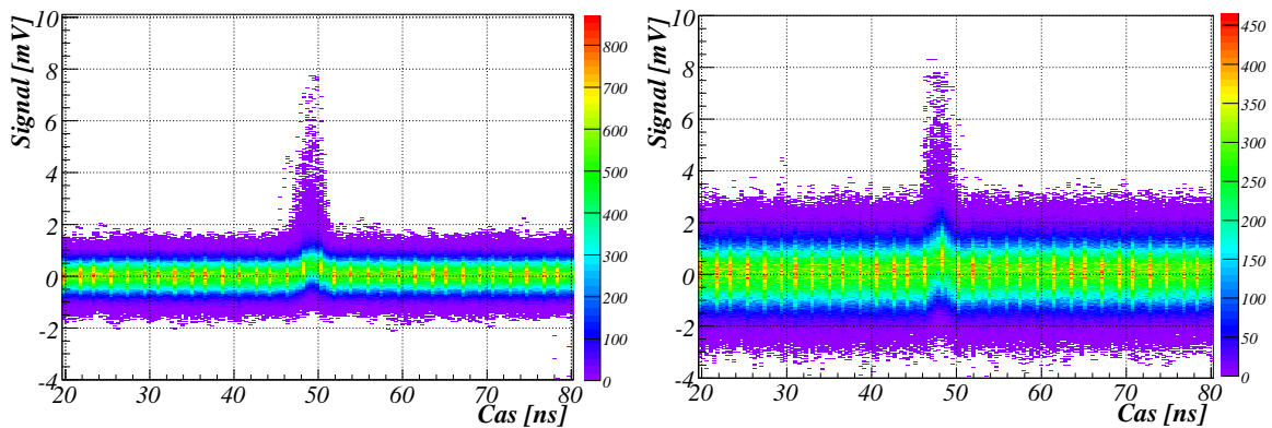
Slika 7.16: Dvovimenzionalni histogram časovnih potekov vseh dogodkov zajetih s 50\ \mu\text{m} epi diodo pri zaporni napetosti 450 V ter frekvenčni pasovni širini 200 MHz (levo) in 1 GHz na bralnem osciloskopu.
