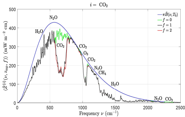
Slika 8: Prikaz enačbe (11) v grafični obliki.
