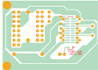
Top Layer (2) Top Silk Screen (255)
