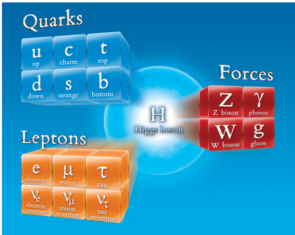
Slika 2: Gradniki Standardnega modela. Delci snovi, kvarki in leptoni, nastopajo v parih treh generacij, ki se razlikujejo po masi. Posredniki sil so gluoni za močno, bozona W in Z za šibko ter foton za elektromagnetno. Vse povezuje Higgsov bozon, ki delcem preskrbi maso.
