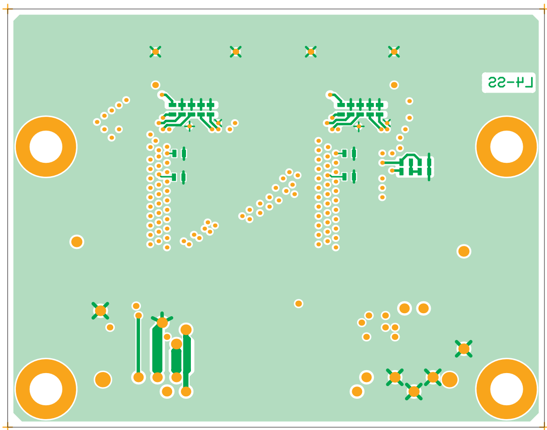
Bottom Layer
