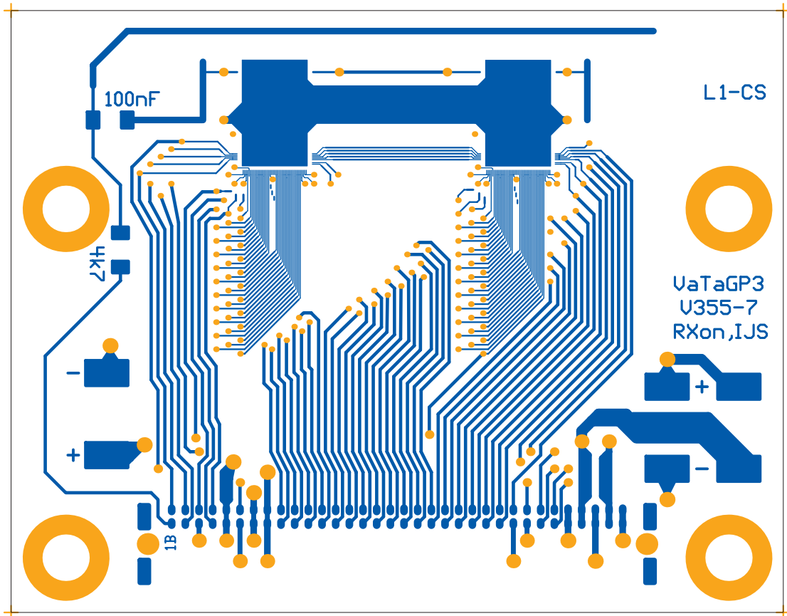
Top Layer
